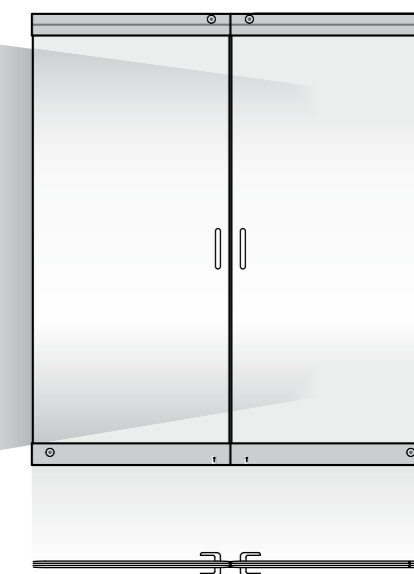
DTZ Dveřní modul (dvoukřídlé dveře) Dva normální panely mohou být nahrazeny dvoukřídlým dveřním panelem. V jakékoliv poloze stěny.
